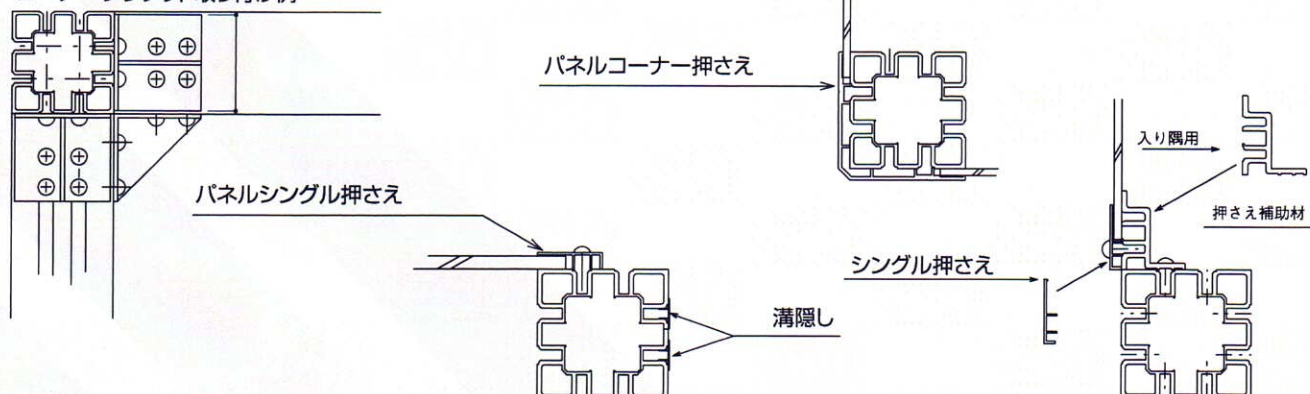
コーナーブラケット取り付け例
